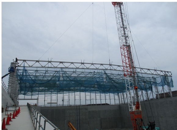
鉄骨工事
